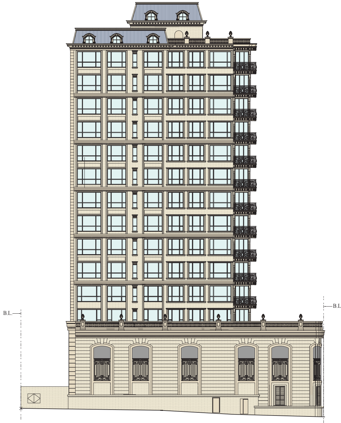
東南面立面圖 SOUTH EAST ELEVATON
