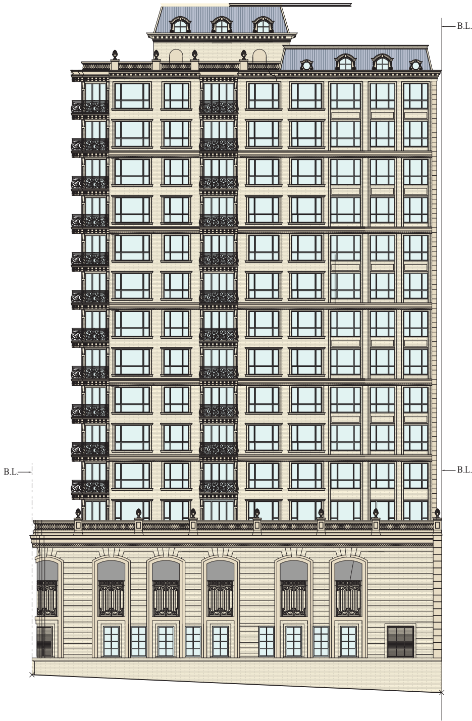
東北面立面圖 NORTH EAST ELEVATON
